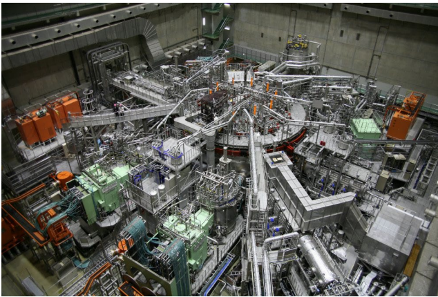
図3 核融合科学研究所 (NIFS) 大型ヘリカル装置 『LHD』・岐阜県土岐市
