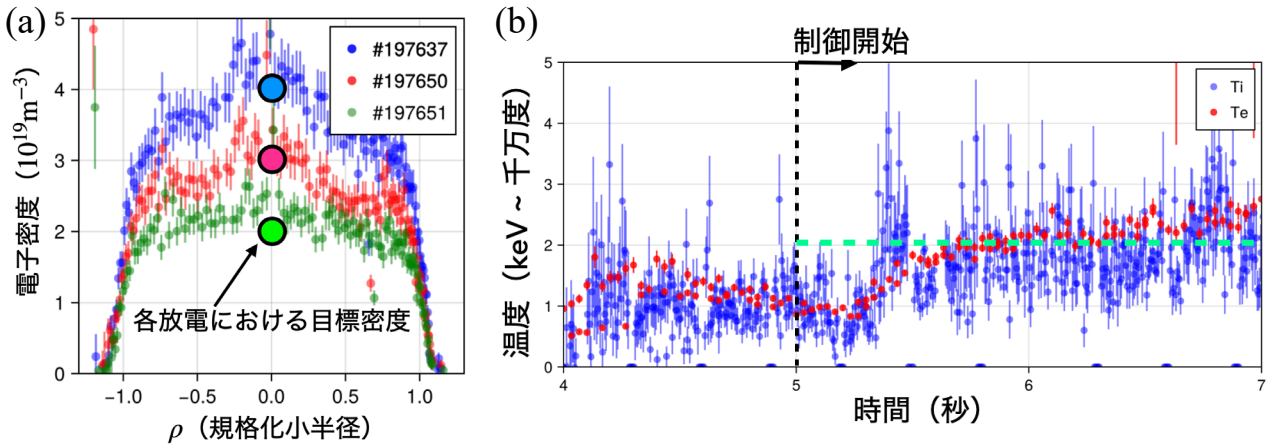
図2 (a)ASTIにより遠隔制御した電子密度分布。 \rho は規格化小半径であり、0がプラズマの中心、 \pm 1 がプラズマの端に対応する。(b)プラズマの中心付近での電子温度 (Te) とイオン温度 (Ti) の時間発展 (#197650)。どちらも 2 keV (約 2 千万度) 付近に制御されている。
