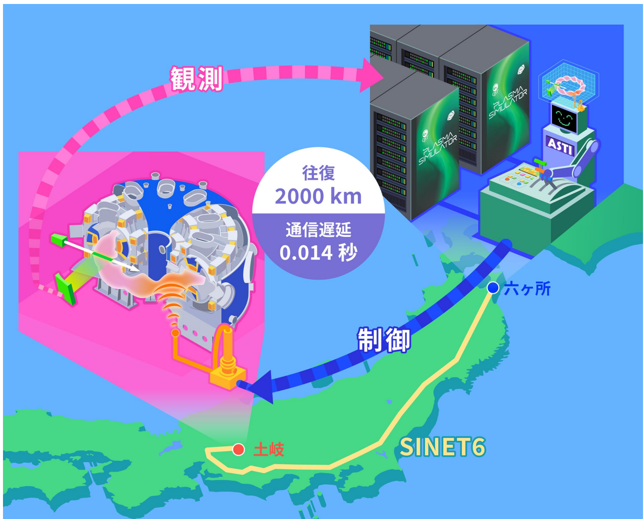
図1 核融合科学研究所(NIFS)の大型ヘリカル装置LHD(岐阜県土岐市)と、NIFSと量子科学技術研究開発機構(QST)が共同調達した新型スーパーコンピュータ”プラズマシミュレータ”(青森県六ヶ所村)を高速学術情報ネットワークSINET6を通して接続したデジタルツイン制御を実現。
