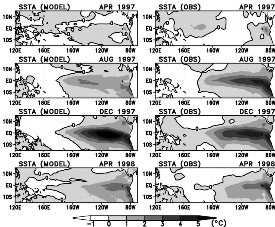
図 2. 熱帯太平洋の予測の例．海面水温の気候値からの偏差の水平分布を、予測結果(左列の図)と同じ時期の観測結果(右列の図)で示す．時期は上から 1997 年 4, 8, 12, 1998 年 4 月である．
