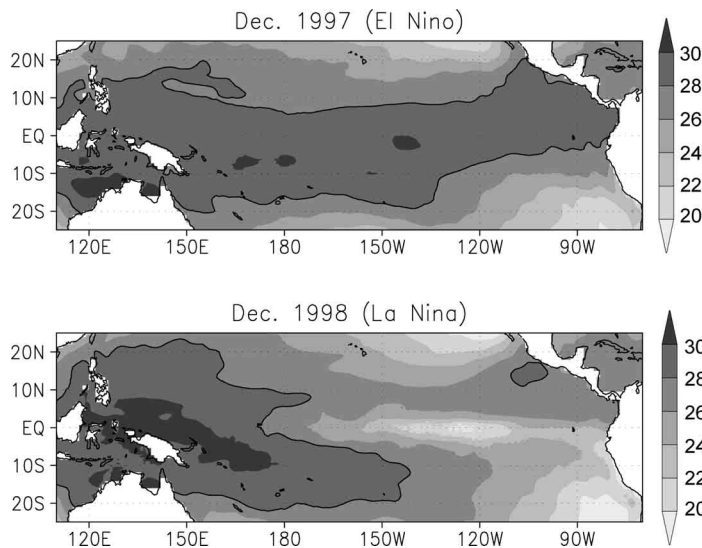
図 1. 海面水温分布．上図：エルニーニョの時期(1997 年 12 月)．下図：ラニーニャの時期(1998 年 12 月)．等値線は 28 度 C の等温線を表す．
