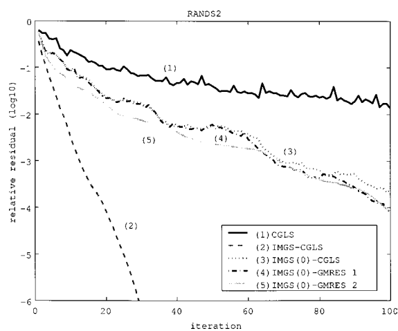
図 1. 反復数 vs. \|A^T r\|_2 / \|A^T b\|_2 (RANDS2).
