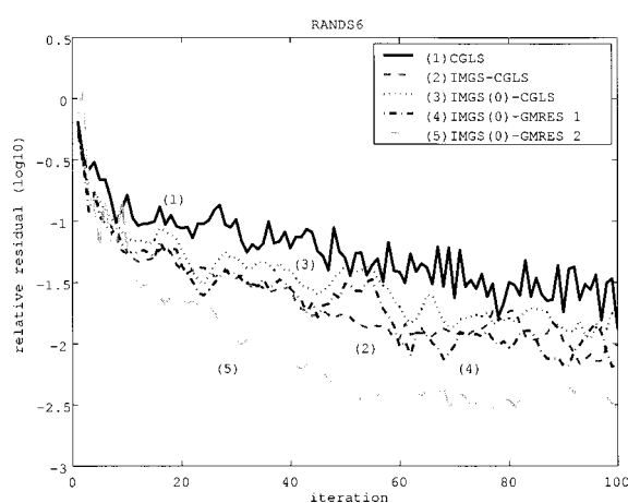
図 2. 反復数 vs. \|A^T r\|_2 / \|A^T b\|_2 (RANDS6).
