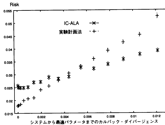
図8. リスクのプロット: IC-ALA, 通常の実験計画法のそれぞれのリスクを標準誤差とともにプロットしたグラフ。横軸はシステムから最適パラメータまでのカルバック・ダイバージェンス。エラーバーは標準誤差を表している。
