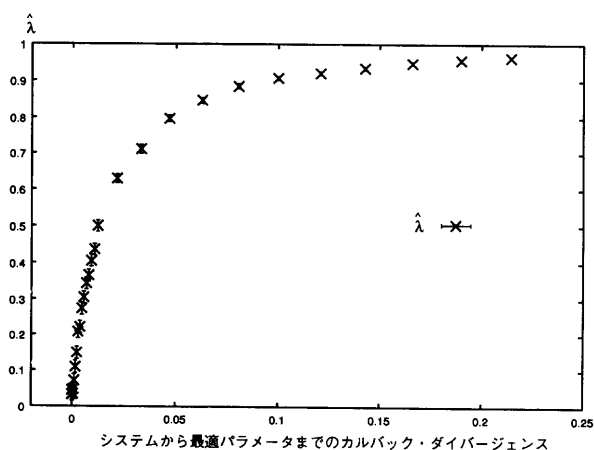
図6. IC-ALAのStep3における \hat{\lambda} の期待値をプロットしたグラフ。横軸はシステムから最適パラメータまでのカルバック・ダイバージェンス。エラーバーは標準誤差を表している。
