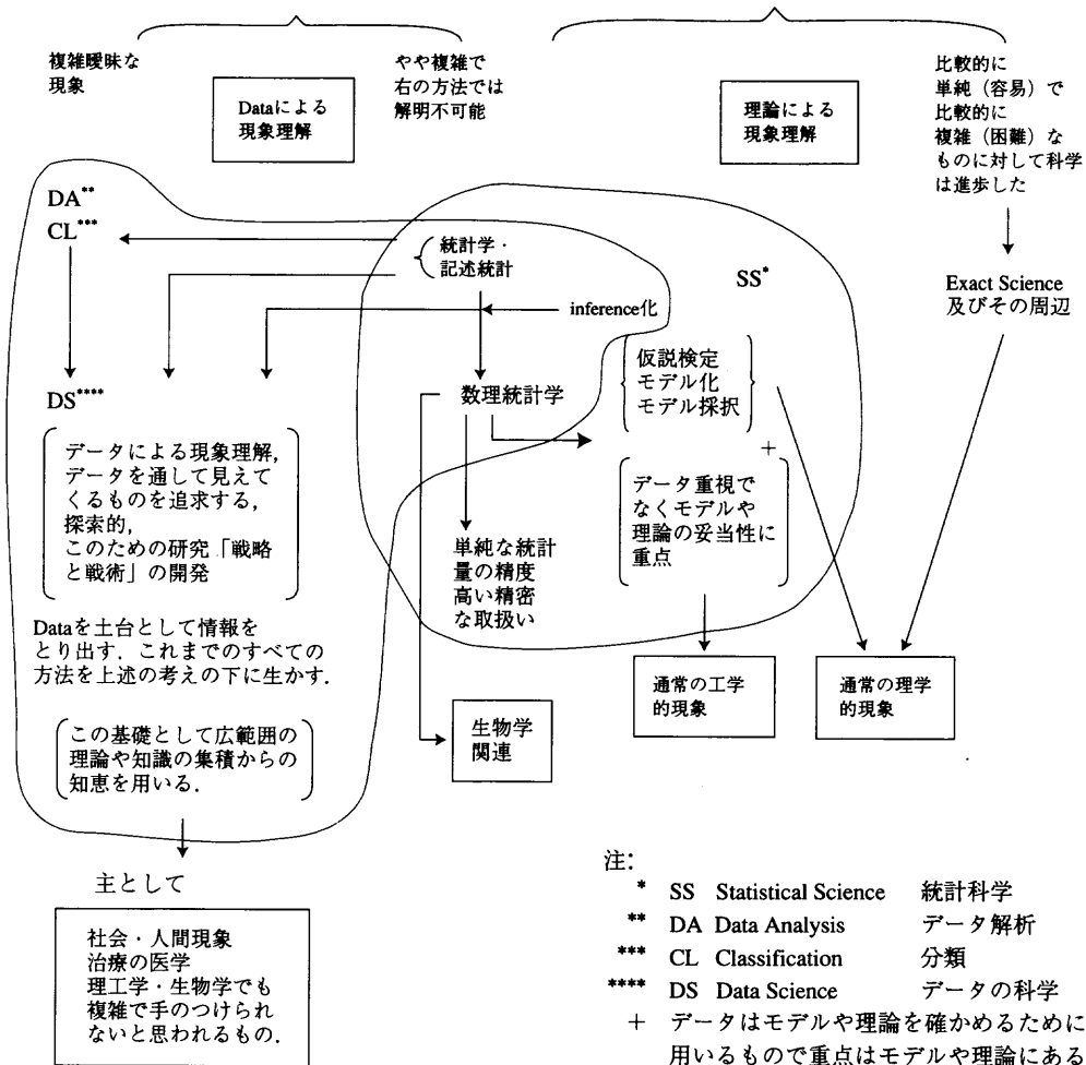
図5. 科学的方法論の中の統計的方法.
