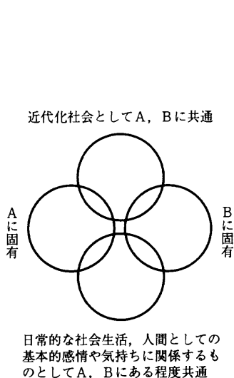
図3. 連鎖的調査計画 — 質問項目の選択。
