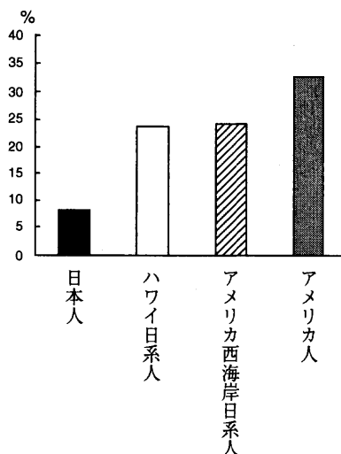
図 32. 義理人情スケール値 0 の比率。
