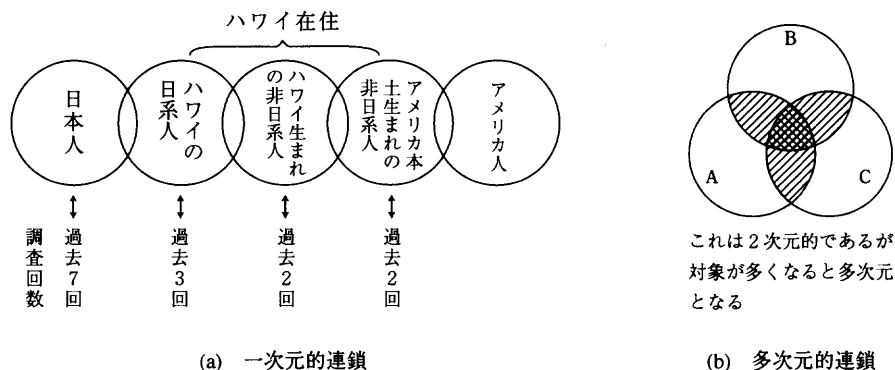
図2. 連鎖的調査計画——調査対象集団の連鎖。
