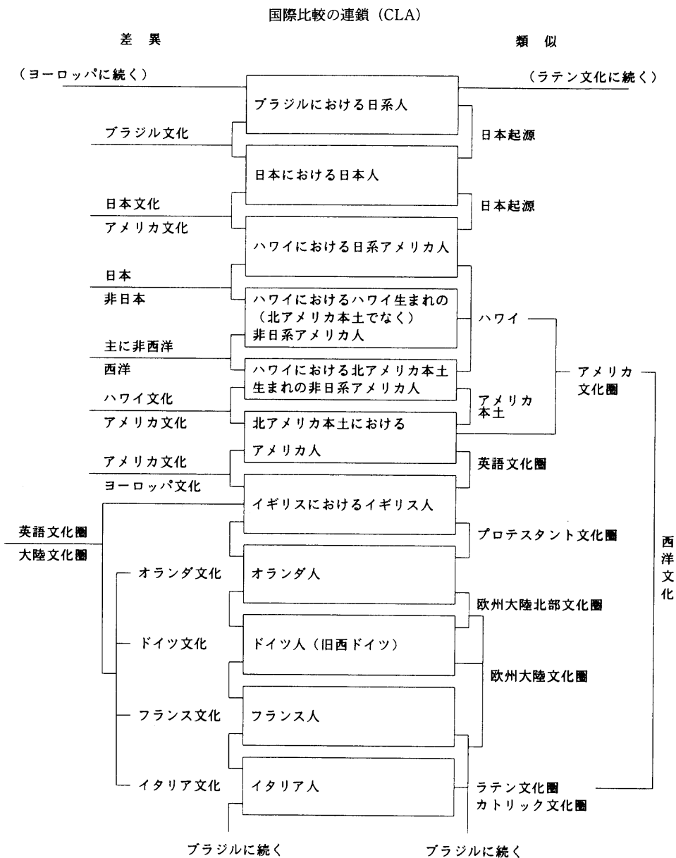
図 22. CLA による対象国：民族。
