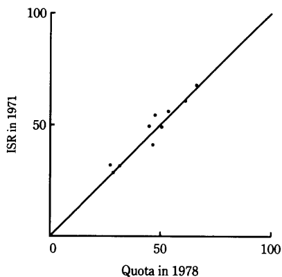
図 15. ランダム・サンプルとクォータ・サンプル。
