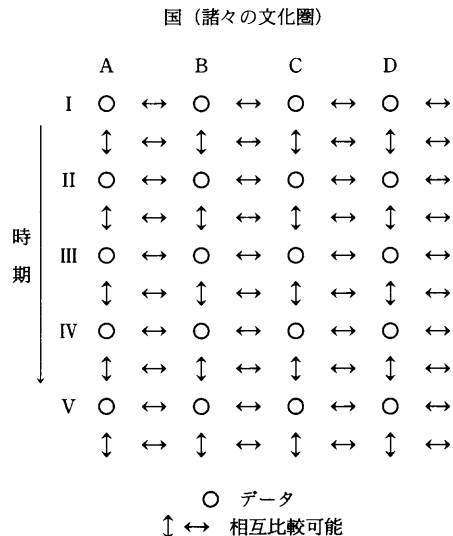
図4. 時間的・空間的連鎖の比較。
