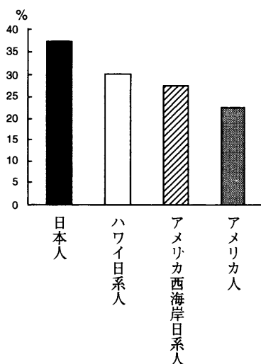
図 33. 人情スケール値 5 以上の比率。
