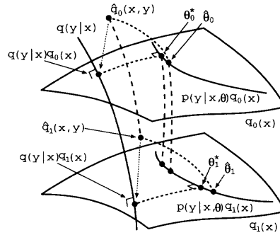
図4. 重み付き MLE の幾何的解釈 (Shimodaira (1998 b)). データを表す経験分布 \hat{q}(y, z) からモデル多様体 \{p(y|z, \theta) q_0(z) : \theta \in \Theta\} に射影した点が MLE \hat{\theta} の予測分布. 経験分布を重み関数 w(z) でシフトした \hat{q}_w(y, z) \propto w(z) \hat{q}(y, z) からモデルに射影したのが, 重み付き MLE \hat{\theta}_w の予測分布. 特に w_1(z) を重み関数に選んだものを, \hat{q}_1(y, z) , \hat{\theta}_1 等と書く. この図で, q_0(z) は多様体 \{q_x(y, z) : \int q_x(y, z) dy = q_0(z)\} を表し, q(y|z) は多様体 \{q_x(y, z) : \int q_x(y, z) dy = q(y|z)\} を表す. q_0(z) と q(y|z) は互いに直交している. 計量が各 foliation q_i(z) で異なることより, 一般に \hat{\theta}_0 \neq \hat{\theta}_1 である.
