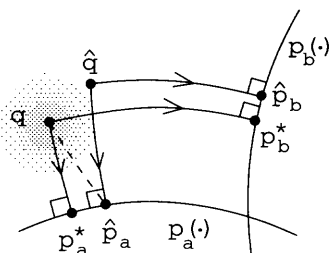
図1. 確率分布の空間におけるMLEなどの幾何的解釈 (Amari (1985)). 各点は x の確率分布を表す. モデルのパラメタを可能な範囲で動かすと点の集合ができるが, それは多様体 (曲面) によって表される. この図では互いにネストの関係にない二つのモデル p_a(x|\theta_a) と p_b(x|\theta_b) がある. 真の分布 q = q(\cdot) からモデルを表す多様体 p_a(\cdot) = \{p_a(\cdot|\theta_a): \theta_a \in \Theta_a\} に射影した点 p_a^* = p_a(\cdot|\theta_a^*) が, モデルの中でもっとも q に近い点である. 射影は, K-L 情報量 D(q; p_a(\theta)) の最小化として定義される. 一方, \hat{q} はデータを表す経験分布で, これからモデル p_a(\cdot) に射影した点 \hat{p}_a = p(\cdot|\hat{\theta}_a) がMLEに相当する予測分布である. 真の分布 q からの予測分布 \hat{p}_a の隔たりを D(q; \hat{p}_a) で測ると, AIC は (モデルによらない定数項と定数倍を除いて) その期待値の推定量になる.
