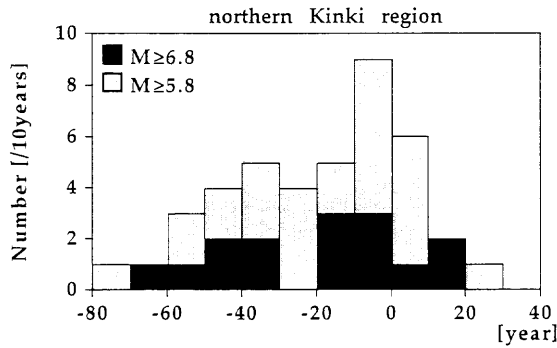
図4. 南海トラフの巨大地震(図の横軸0)前後の近畿中北部の大地震の活動。10年ごとの数を8回の巨大地震で重ねさせてある。
