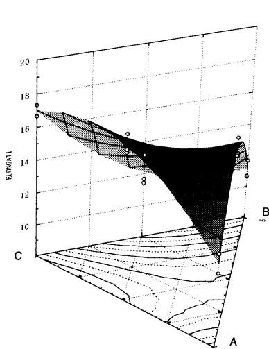
図8. 応答曲面の3次元グラフ。
