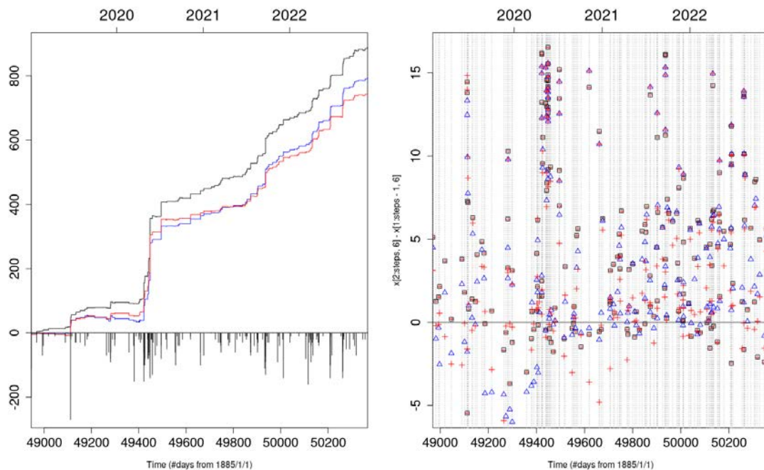
第 2 図 各種時空間 ETAS モデルの (左図) 対数尤度スコア (2) と (右図) それらの差分 (3) の時間的推移。
