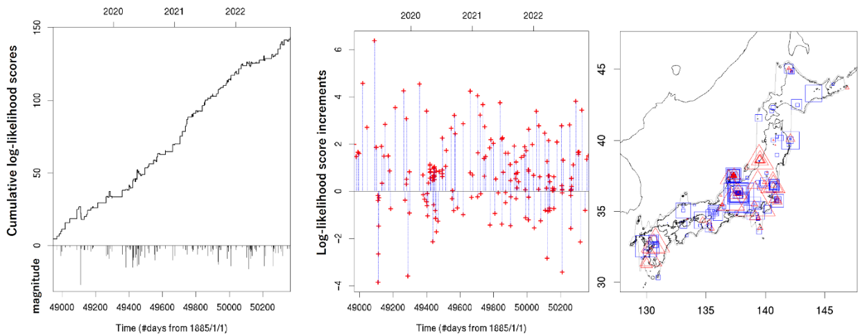
第4図 HIST-ETAS5pa (a) モデルの通常時空間 ETAS (c) モデルに対する対数尤度スコアの比較。
