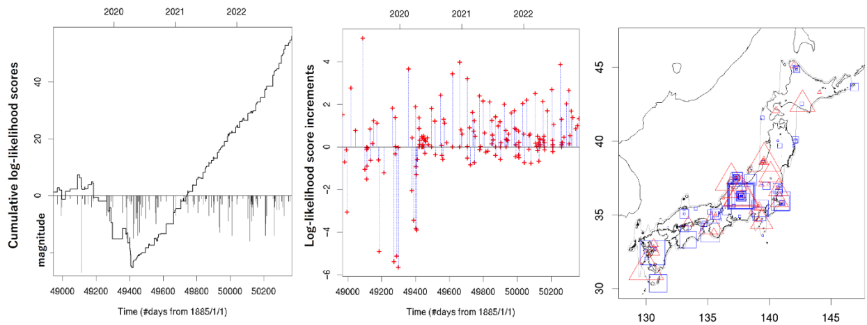
第3図 HIST-ETAS- \mu K (b) モデルの通常時空間 ETAS (c) モデルに対する対数尤度スコアの比較。
