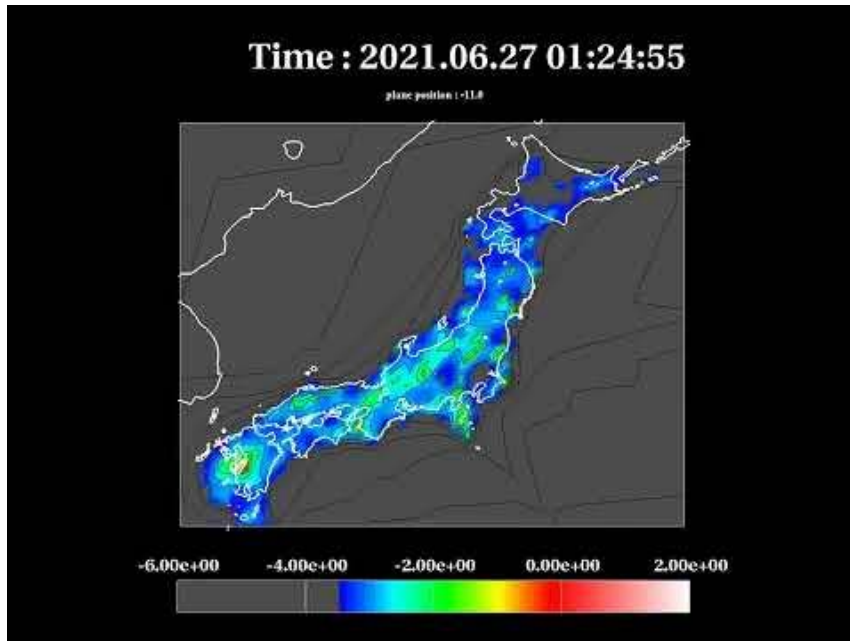
第 1 図 HIST-ETAS5pa (a) モデルの短期予測の動画
