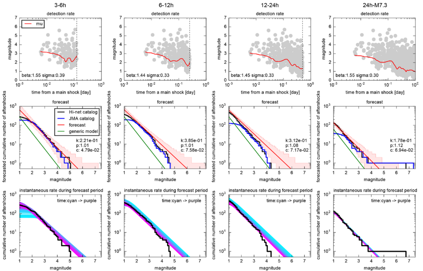
第1図. 2016/04/14 の熊本の地震 (M6.5, 前震) 後の本震発生までの地震活動の確率予測。予測モデルとして大森・宇津則と Gutenberg-Richter 則を用い、Hi-net 自動処理震源カタログを用いてパラメータの推定を行った。一番上のパネルはそれぞれの学習期間における余震検出率の推定を表している。真ん中のパネルは予測結果 (赤色) と実際の観測値 (黒: Hi-net カタログ, 青: JMA カタログ) を比較している。参考のために日本の余震活動の平均的なパラメータ値を用いた予測結果 (緑) も示した。一番下のパネルは予測期間における瞬間発生率の時間の変化をプロットしたものである。色は時間を表しており、シアンから紫へと時間が経過する。
