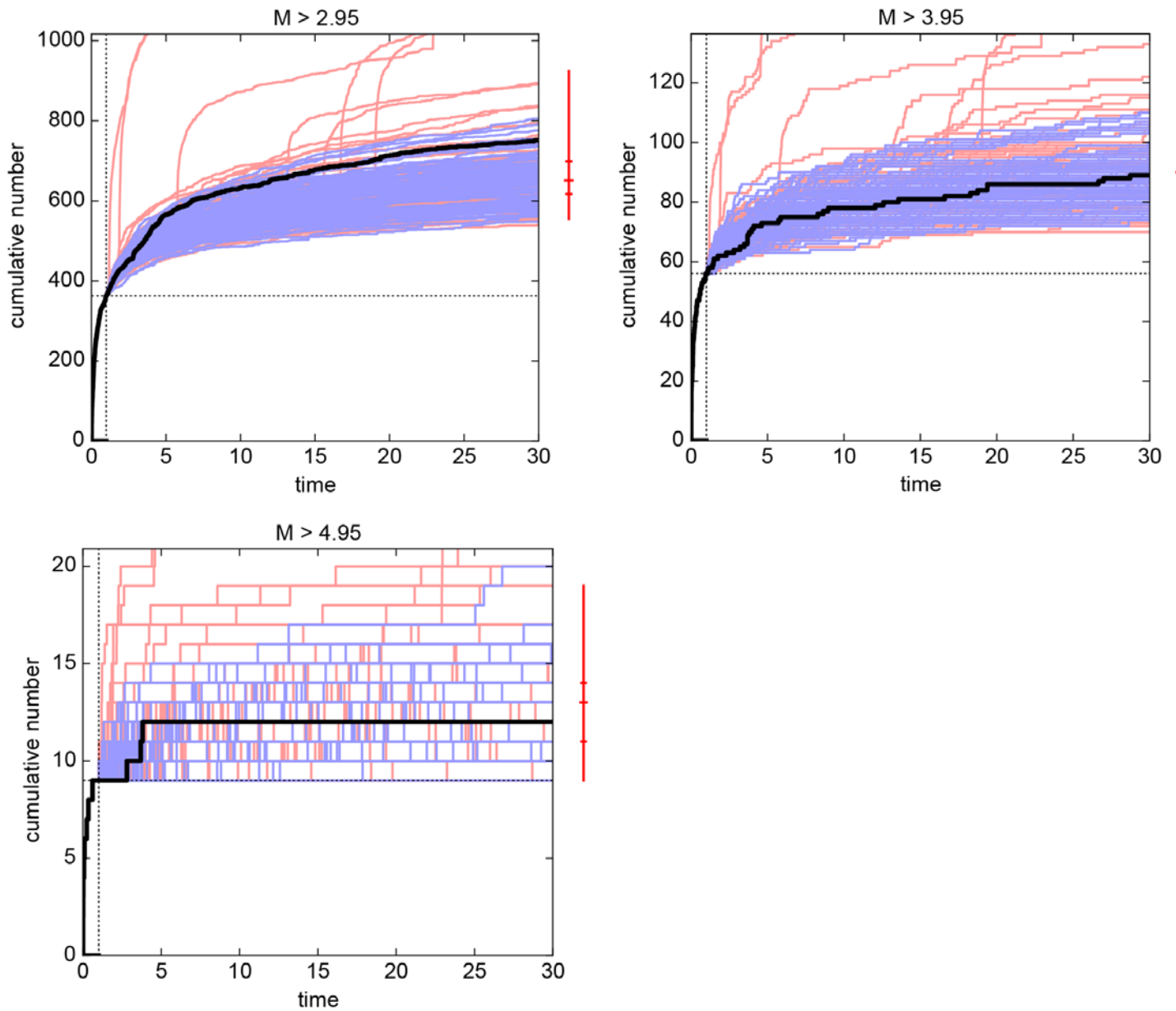
第4図. ETAS モデルを用いた 2016 年熊本地震の本震以降の余震活動の中期予測。本震後 1 日間のデータ (JMA カタログ) から ETAS モデル及び GR 則のパラメータを推定し、その後一ヶ月間の活動の予測をシミュレーションを用いて行った。ETAS モデルのパラメータは事後分布からサンプルされた 1000 のパラメータ値を用い、シミュレーション一回ごとにパラメータ値を変えて予測を行った (ベイズ予測)。マグニチュードの分布としては GR 則を用いているが、青線は学習期間に起きた最大の余震のマグニチュードに 0.3 を足したものよりも大きな余震は起こらないような制限を加えてシミュレーションを行ったものである。赤線は本震と同じマグニチュードまでの余震を許容してシミュレーションを行った結果である。この異なるマグニチュード分布からの予測を組み合わせ得られる予測分布の 2.5%, 25%, 50%, 75%, 97.5% 点を示したものがパネルの右側の赤いバーである。黒線は JMA カタログからの観測値を示している。なお中期予測における ETAS モデルの有用性は 202 回予知連にて報告を行っている。
