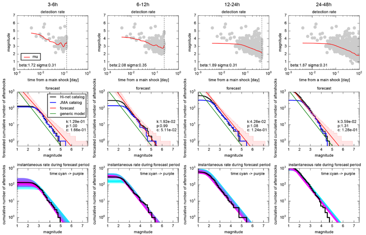
第2図. 2016/04/16の熊本の地震 (M7.3, 本震) 後の余震活動の確率予測。図の様式は第一図と同じ。
