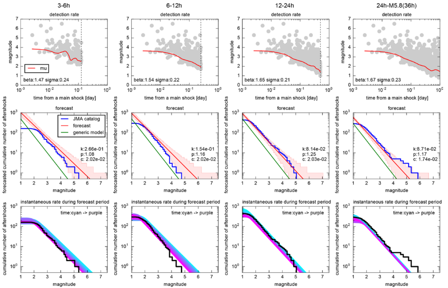
第3図. 2003年新潟県中越地震(M6.8)後の余震活動の確率予測。図の様式は第一図と同じ。ただしここでは予測はJMAカタログを用いて行われている。
