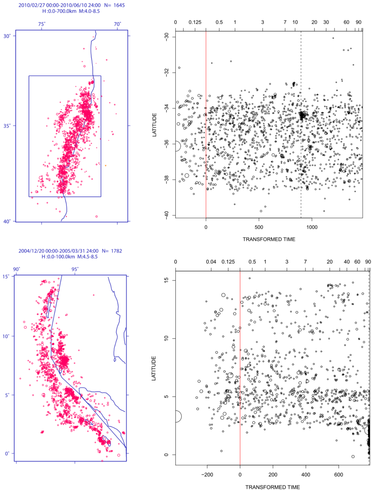
2010年チリ地震（Mw8.8）の余震活動（上図）と2004年スマトラ地震（Mw9.0）のプレート境界部分の余震活動（下図）のデトレンド時空間分布。
