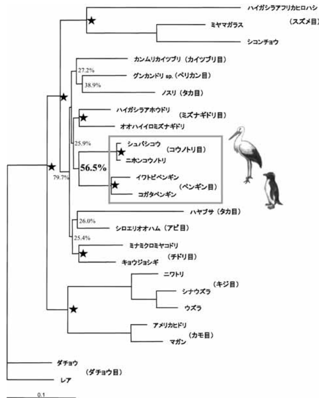
図3. ミトコンドリア全長アミノ酸配列に基づいたML系統樹2. 本解析では7種のアウトグループを使用した. 系統樹中の各ブランチの長さは, アミノ酸変異数の割合に基づいて算出した. クレード上の数値はBP値を示す. 星印はQP法による予備的解析によって単系統性が確実であるとみなされ固定されたクレードを表す.
