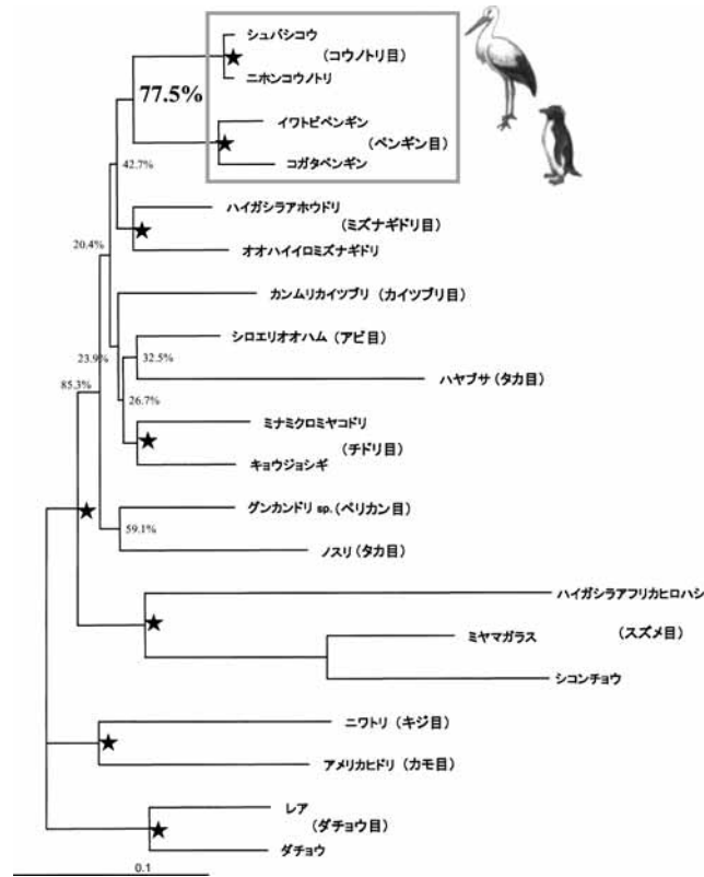
図 2. ミトコンドリア全長アミノ酸配列に基づいた ML 系統樹 1. 本解析では 4 種のアウトグループを使用した. 系統樹中の各ブランチの長さは, アミノ酸変異数の割合に基づいて算出した. クレード上の数値は BP 値を示す. 星印は QP 法による予備的解析によって単系統性が確実であるとみなされ固定されたクレードを表す.
