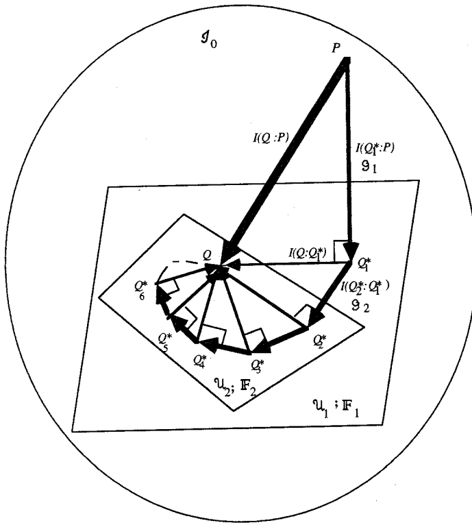
図1. 逐次 Legendre 変換によるモデルの更新.
